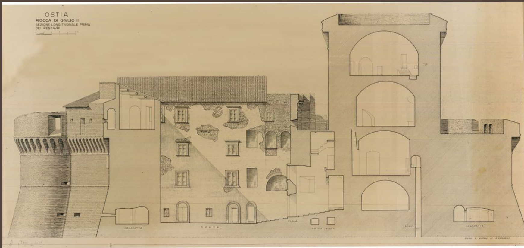
G. Pascolini, Castello di Giulio II: sezione prima del restauro, 1941-42
